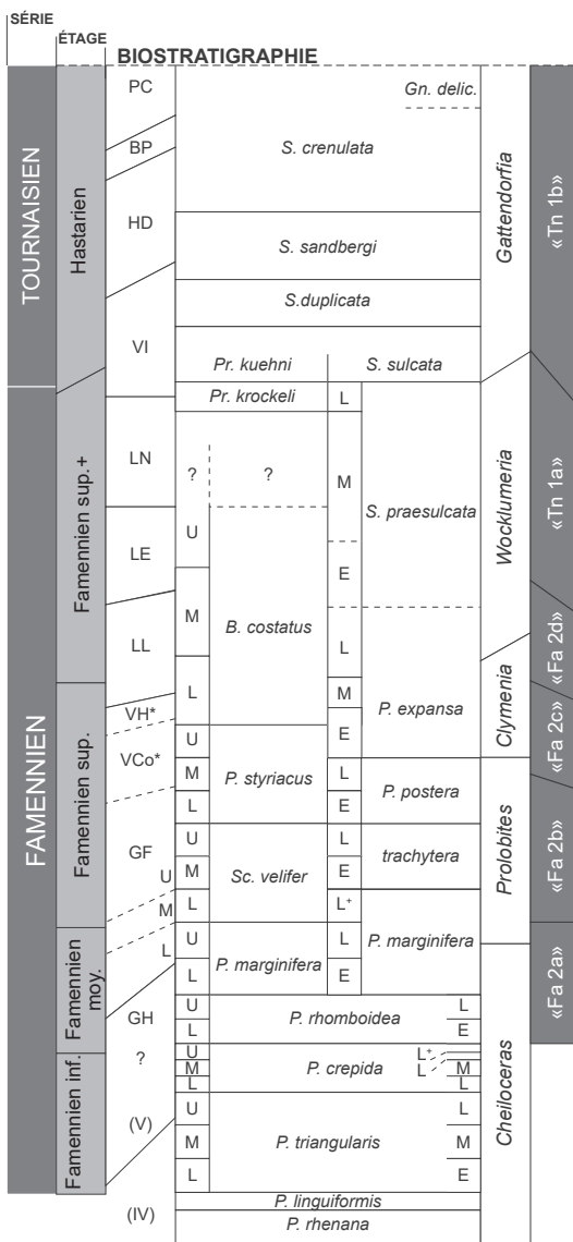
Fig. 7. Cadre biostratigraphique du Famennien et du Tournaisien inf., avec indication, dans la cadre de droite, de l'ancienne subdivision lithostratigraphique belge devenue obsolète (d'après THOREZ et al, 2006).
