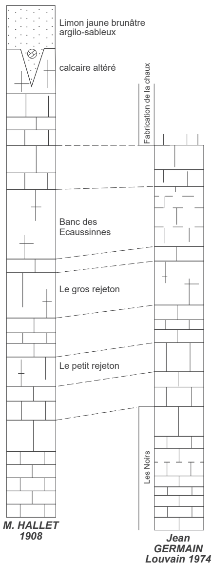
Fig. 22.coupe de la carrière des Nutons avec noms anciens des bancs, donnés par les exploitants de carrières de « Petit Granit » (d'après GROESSENS, 1978).
