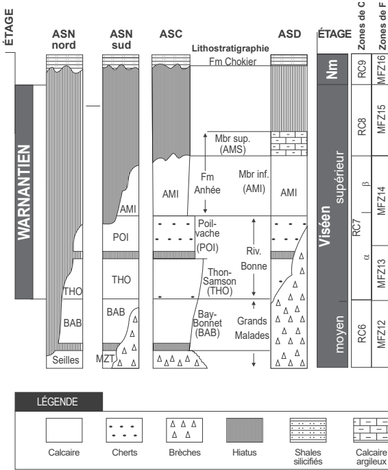
Fig. 18. Schéma biostratigraphique du Warnantien en Belgique (Synclinorium de Dinant), d'après POTY et HANCE (2006).
