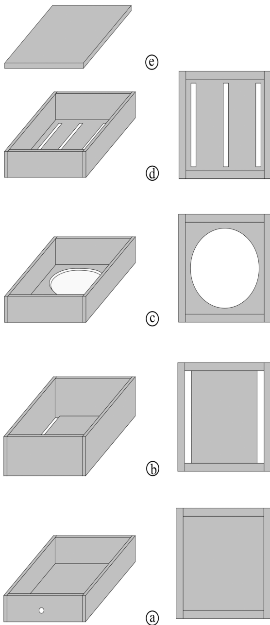
Figure 3: Ruche modifiée de l'Instituto Nacional de Pesquisas da Amazônia (INPA). A gauche une vue en perspective et à droite une vue de dessous des compartiments : a premier compartiment avec un trou d'entrée (45 x 45 x 5 cm) ; b compartiment à couvain (45 x 45 x 12 cm) avec deux ouvertures à la base (40 x 1 cm) ; c compartiment extension du couvain (45 x 45 x 4 cm) avec une ouverture de 35 cm de diamètre à la base ; d compartiment pour pot de pollen et miel (45 x 45 x 7 cm) avec trois ouvertures à la base (40 x 2 cm) ; e toit de la ruche. Les dimensions des compartiments correspondent aux dimensions intérieures.
